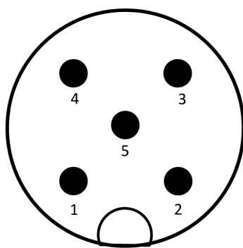
Schemazeichnung M12-Stecker Cross Section M12 connector
