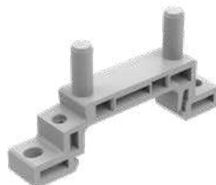
Klemme VC Holder Pin 16 667416-50 (Schraube 3,0x10) für DIN-Schienen Befestigung 201803-1000
