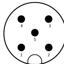
Schemazeichnung M12-Stecker Cross Section M12 connector
